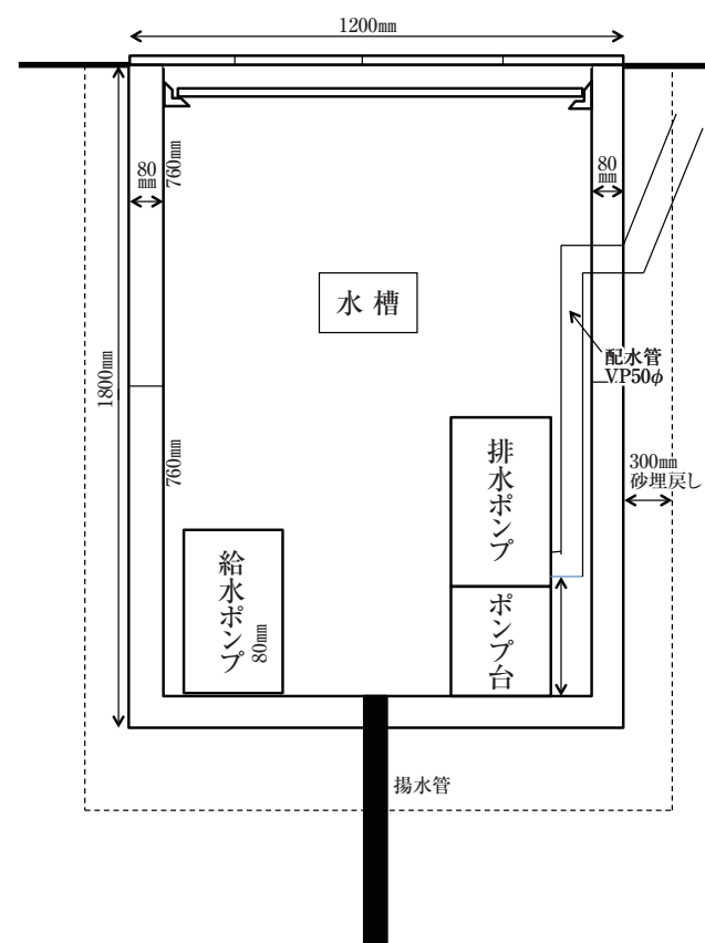
❄️融雪槽断面図❄️
